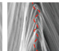
TGテクノロジーを採用して研磨したカミソリの刃の拡大図
